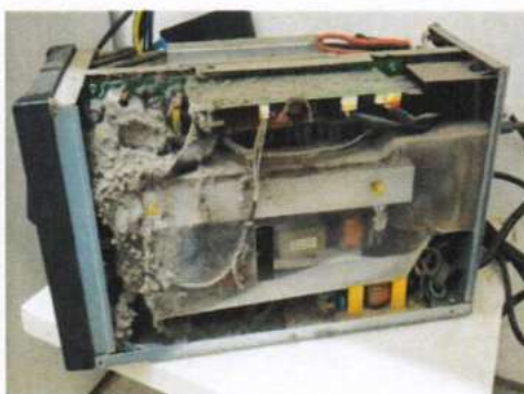
10- PREVENTIVA NOBREAK RAIOS-X
